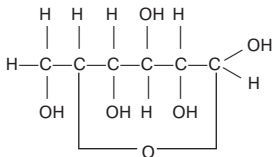
\beta -глюкопираноза
