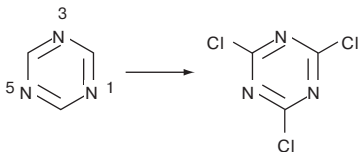
2,4,6-трихлор-1,3,5-триазин (цианурхлорид)
