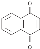
1,4-нафтохинон желтый
