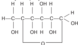
\alpha -глюкопираноза
