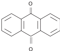
9,10-антрахинон красный
