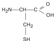
цистеин
